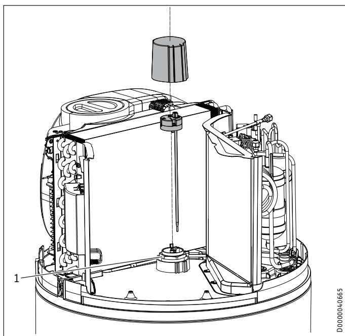
1 Elektrický nouzový/přídavný ohřev s ochrannou anodou
