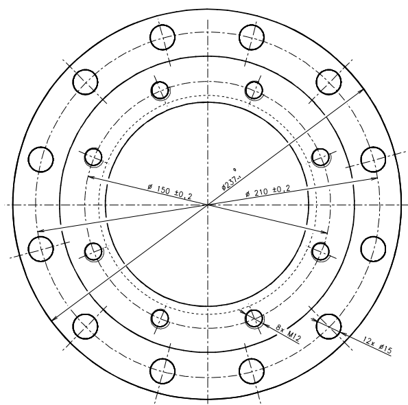
Redukčná príruha 210 / 150
